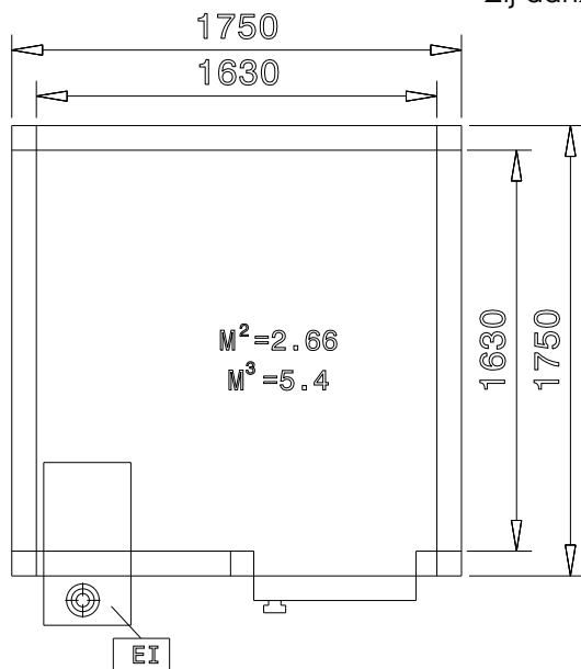
Zij aanzicht
